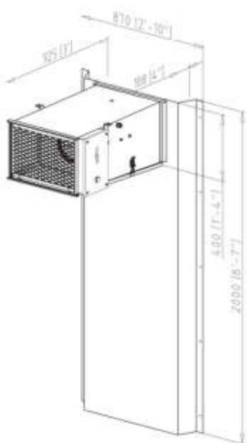
ZVLHČOVAČ EB-10
