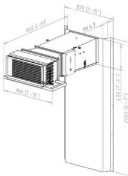
ZVLHČOVAČ EBK-10
