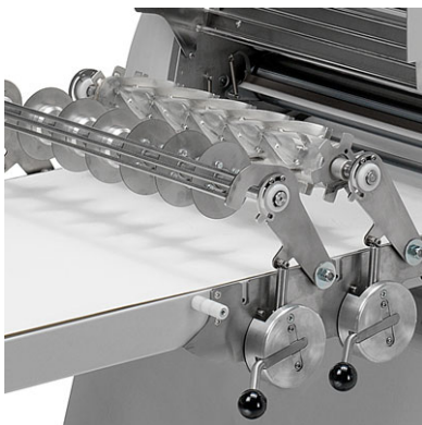
Řezací zařízení s válečky – volitelná výbava všech modelů
